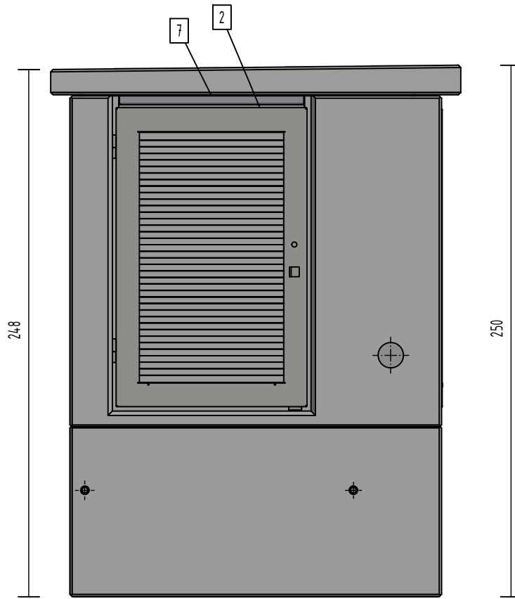
Ansicht B
