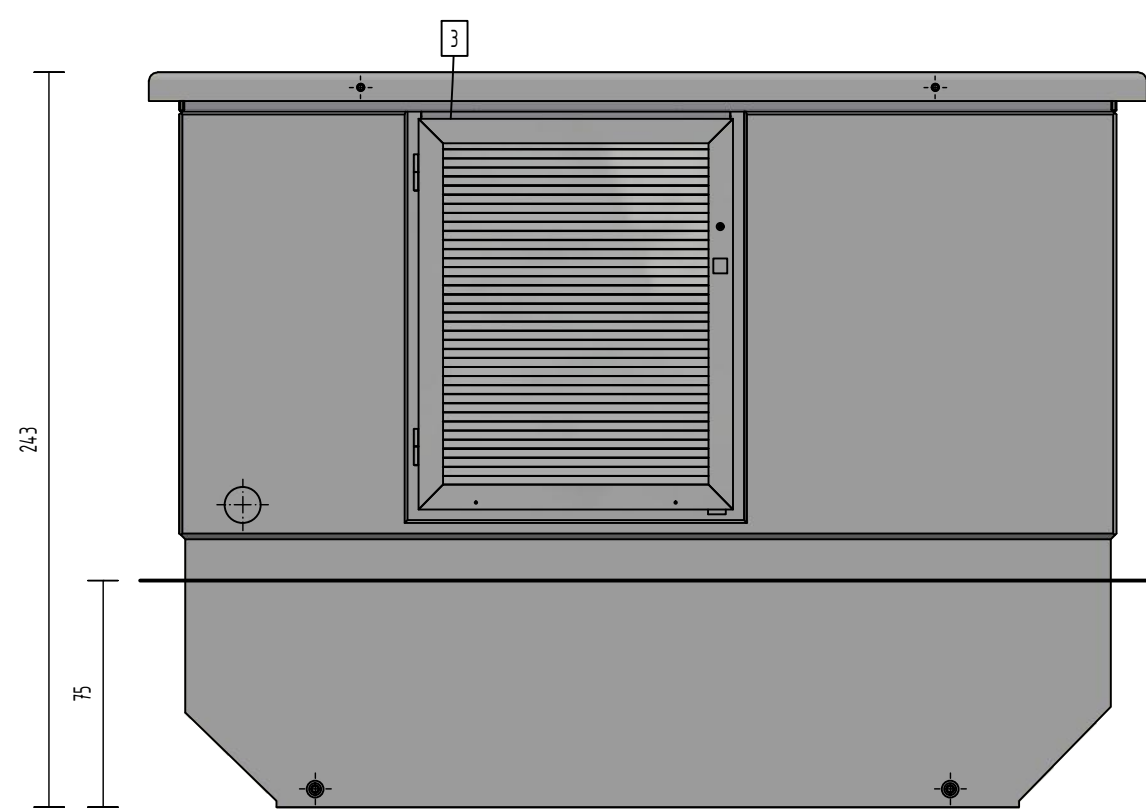
Ansicht A
