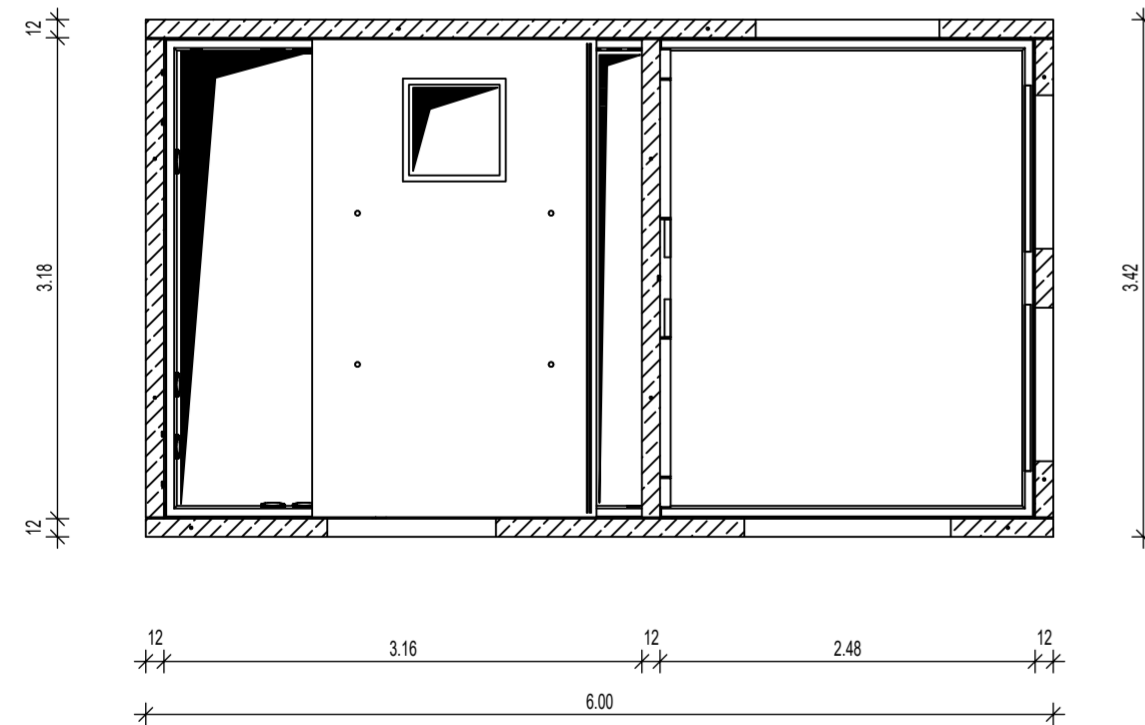
Grundriss
