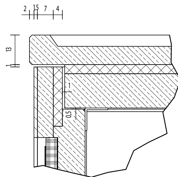
Detail A ( 1 : 10 ) Dachaufkantung
