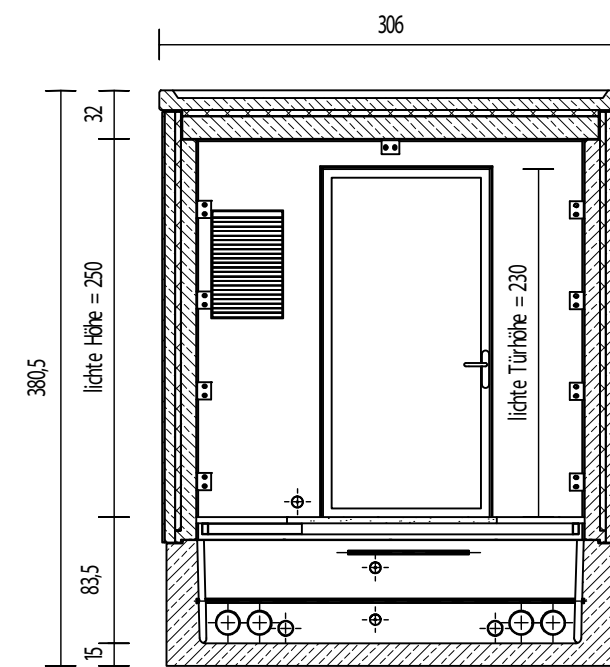
Schnitt A-A
