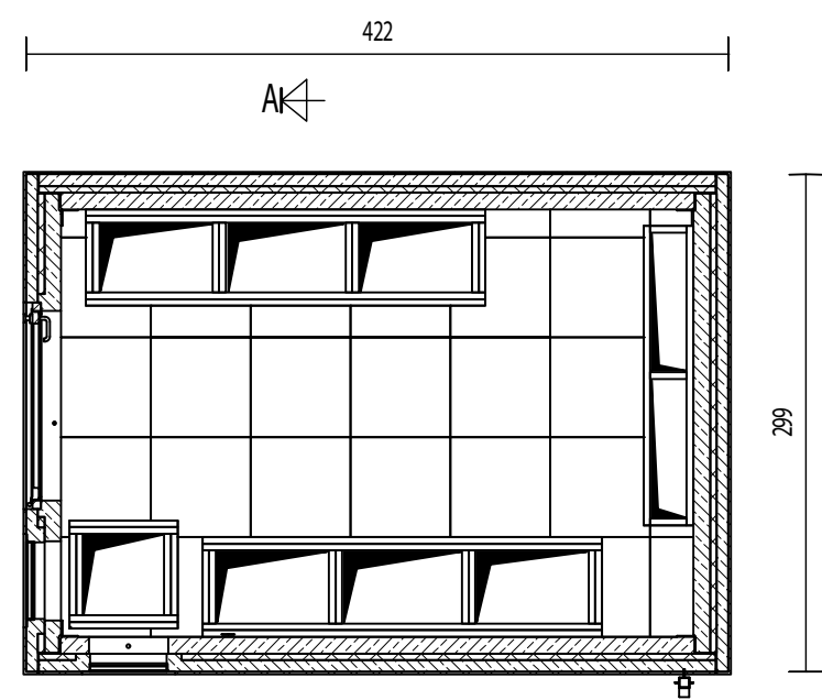
Grundriss
