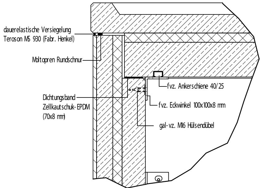
Detail A ( 1 : 10 ) Dachaufkantung
