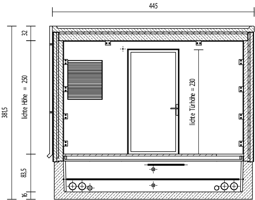
Schnitt A-A
