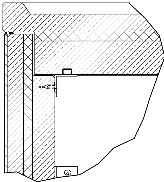
Detail A ( 1 : 10 ) Dachaufkantung
