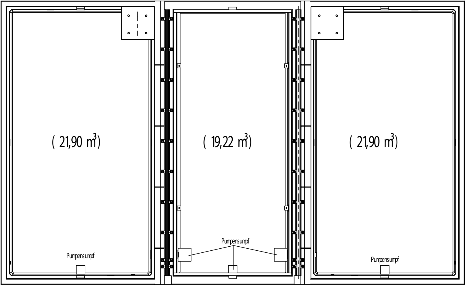
Wännendraufsicht (Ohne Decken und Feuerschutzroste)
