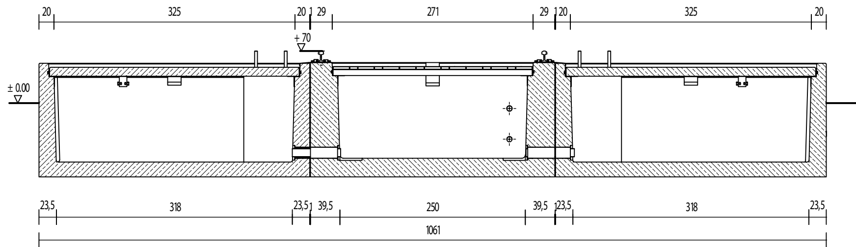
Schnitt
