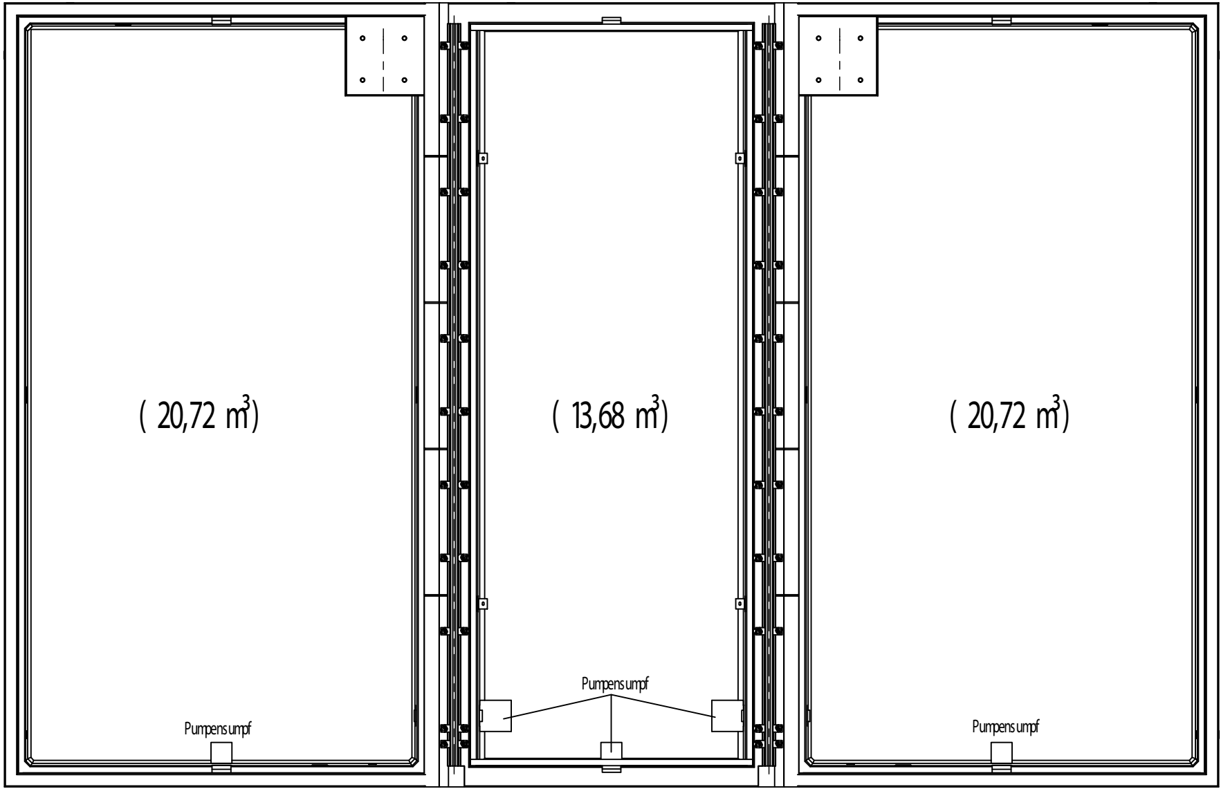
Wannendraufsicht (Ohne Decken und Feuerschutzroste)
