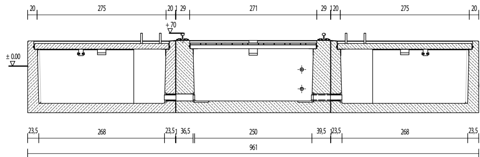
Schnitt
